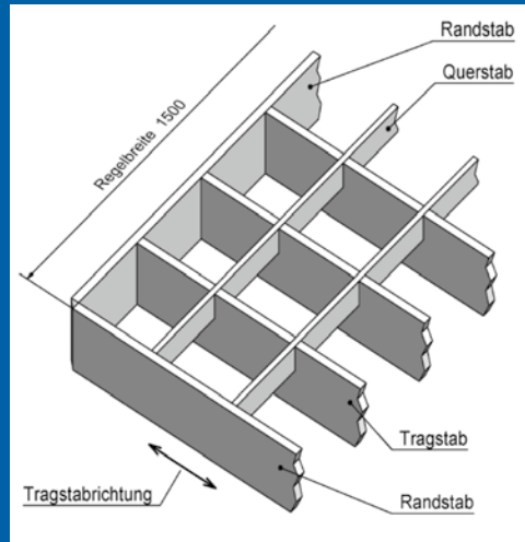
Bild 2: Pressrost
