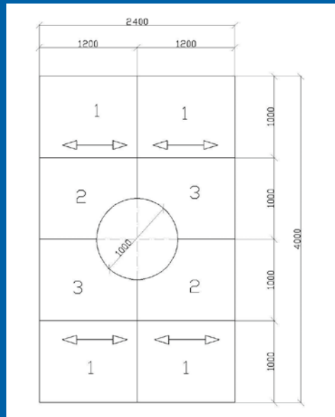
Bild 37: Verlegeplan
