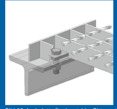
Bild 25: Lochplatte (horizontal im Gitterrost)
