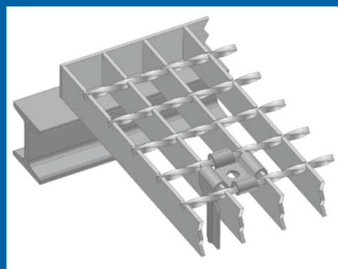
Bild 40: Beispiel einer (nachträglich anzubringen) technischen Maßnahme, die das falsche Einlegen eines quadratischen Gitterrosts verhindert.
