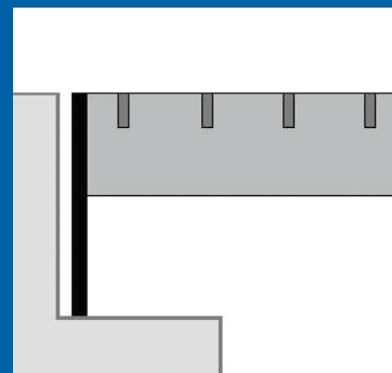
Bild 24: Beispiel einer Aufstelzung
