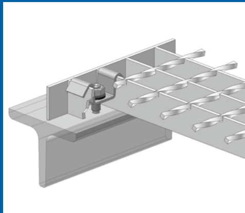
Bild 44: Schweißbolzenbefestigungen
