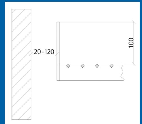
Bild 48: Zusätzliche Schutzmaßnahme (Fußleiste) bei einem Abstand zu angrenzenden Bauteilen > 20 ≤ 120 mm.
