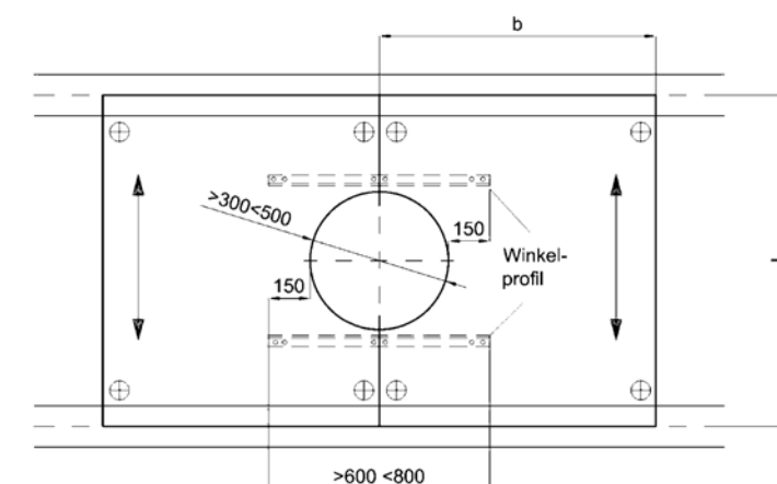
Bild 54: Kreisförmiger Ausschnitt ( > 300 mm < 500 mm) zwischen zwei Gitterrosten (symmetrische Lage) mit Winkelprofil Verbindung zwischen den Gitterrosten (bei mittiger Lage)
