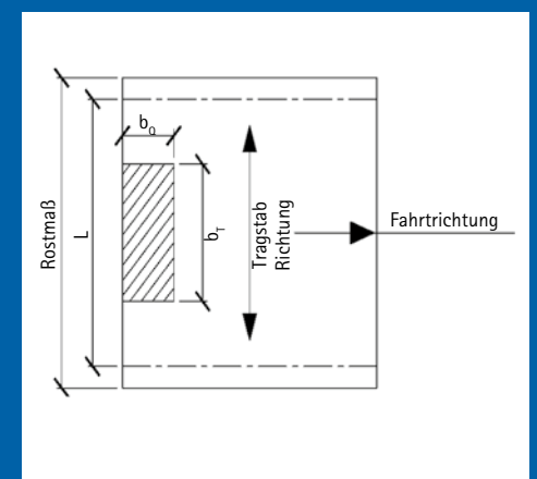
Bild 11: Lastanordnung 1
