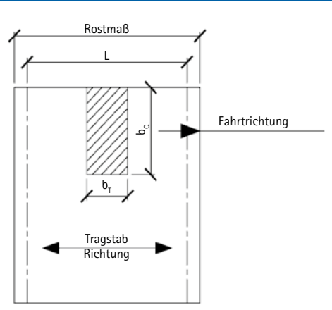
Bild 12: Lastanordnung 2
