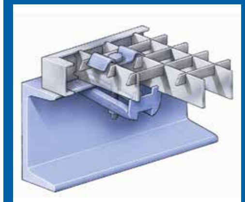
Bild 41: Standardbefestigung – Abhebesicherung
