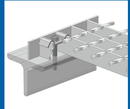
Bild 47: selbstbohrende Schrauben
