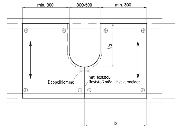
Bild 52: U-förmiger Ausschnitt ( > 300 mm \leq 500 mm) zwischen zwei Gitterrosten mit Doppelklemmenbefestigung (bei Gitterrosttrennung)
