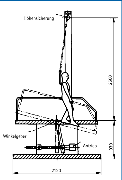
Bild 16: Prüfvorrichtung zur Ermittlung der Rutschhemmung
