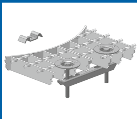
Bild 46: Doppelklemmenbefestigungen
