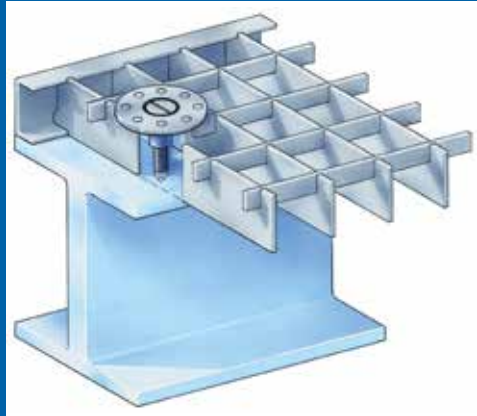
Bild 43: Setzbolzenbefestigung
