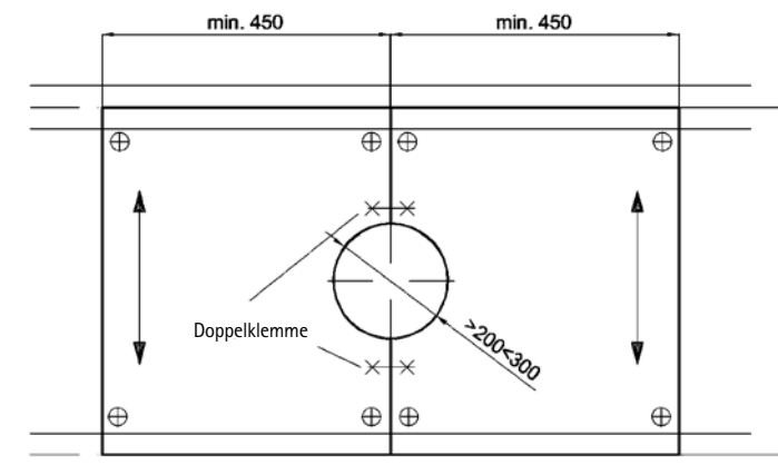
Bild 53: Kreisförmiger Ausschnitt ( > 200 mm < 300 mm) zwischen zwei Gitterrosten (symmetrische Lage) mit Doppelklemmenbefestigung (bei mittiger Lage)
