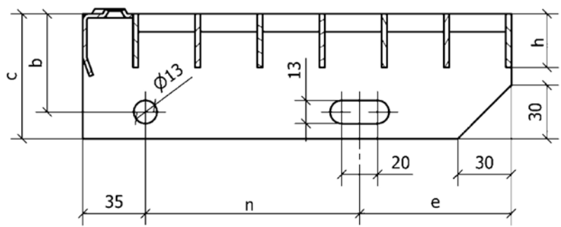
Bild 29: Bild einer Treppenstufe mit Seitenplattendetails (zeichnerischer Schnitt)
