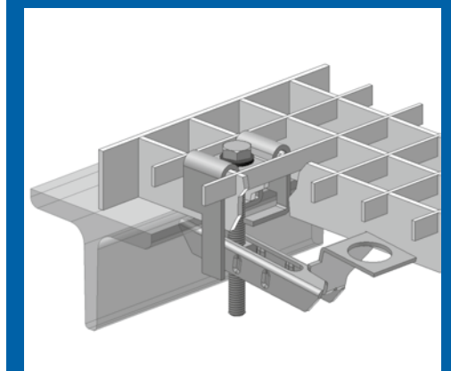
Bild 42: Beispiel einer Sicherheitsbefestigung an einem Pressrost
