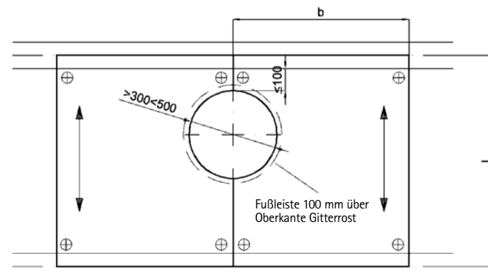
Bild 56: Kreisförmiger Ausschnitt (> 300 mm < 500 mm) zwischen zwei Gitterrosten (asymmetrische Lage) mit Fußleiste (bei Lage nahe der Unterstüztung)
