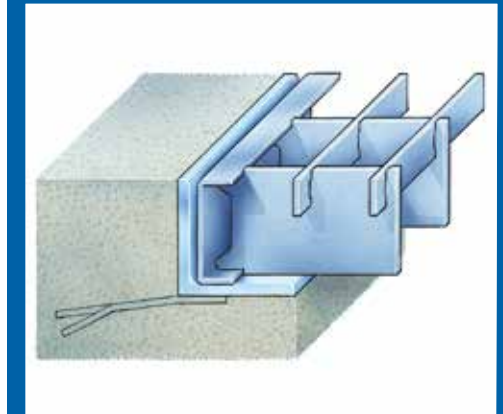
Bild 32: Darstellung einer Gitterrostauflage im Winkelrahmen
