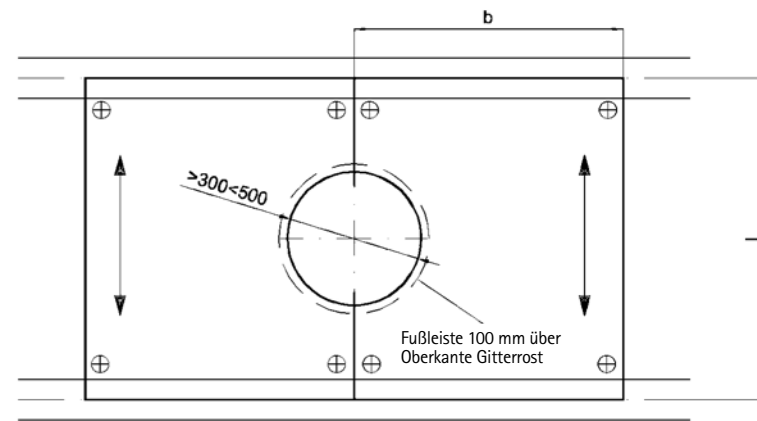
Bild 55: Kreisförmiger Ausschnitt (> 300 mm < 500 mm) zwischen zwei Gitterrosten (symmetrische Lage) mit Fußleiste (bei mittiger Lage)
