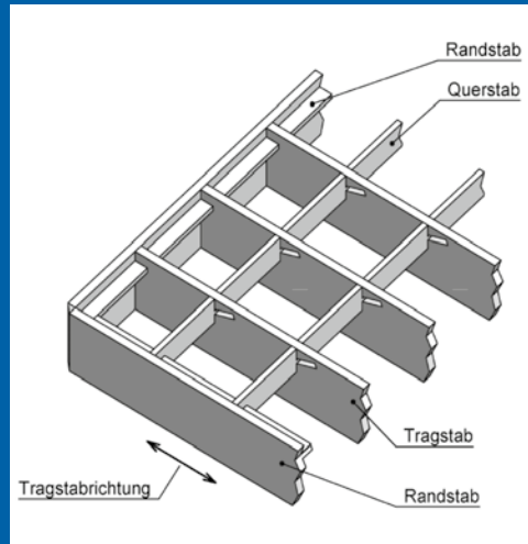
Bild 3: Steckrost
