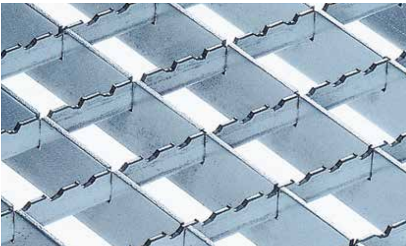
Bild 14: Gitterrost mit Ausnehmungen im Querstab
