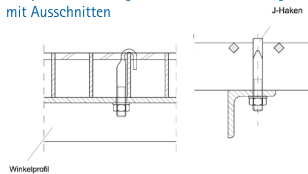
Bild 58 und 59: J-Haken
