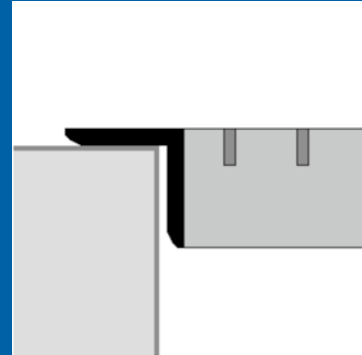
Bild 19: Einhängewinkel (Winkelkragen)
