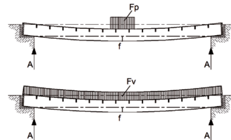
Bild 8: statisches System
