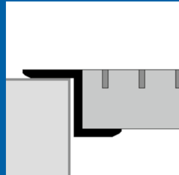
Bild 20: Einhängewinkel (Z-Kragen)
